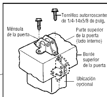
PUERTA METÁLICA
