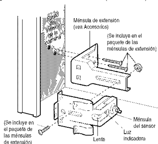
Figura 3 INSTALACIÓN EN LA PARED (LADO DERECHO)
